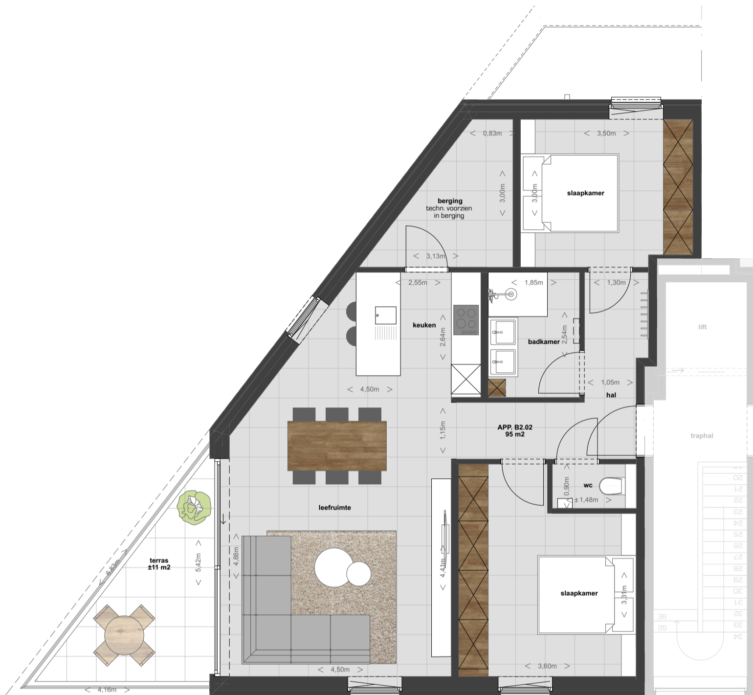
1e VERDIEPING
